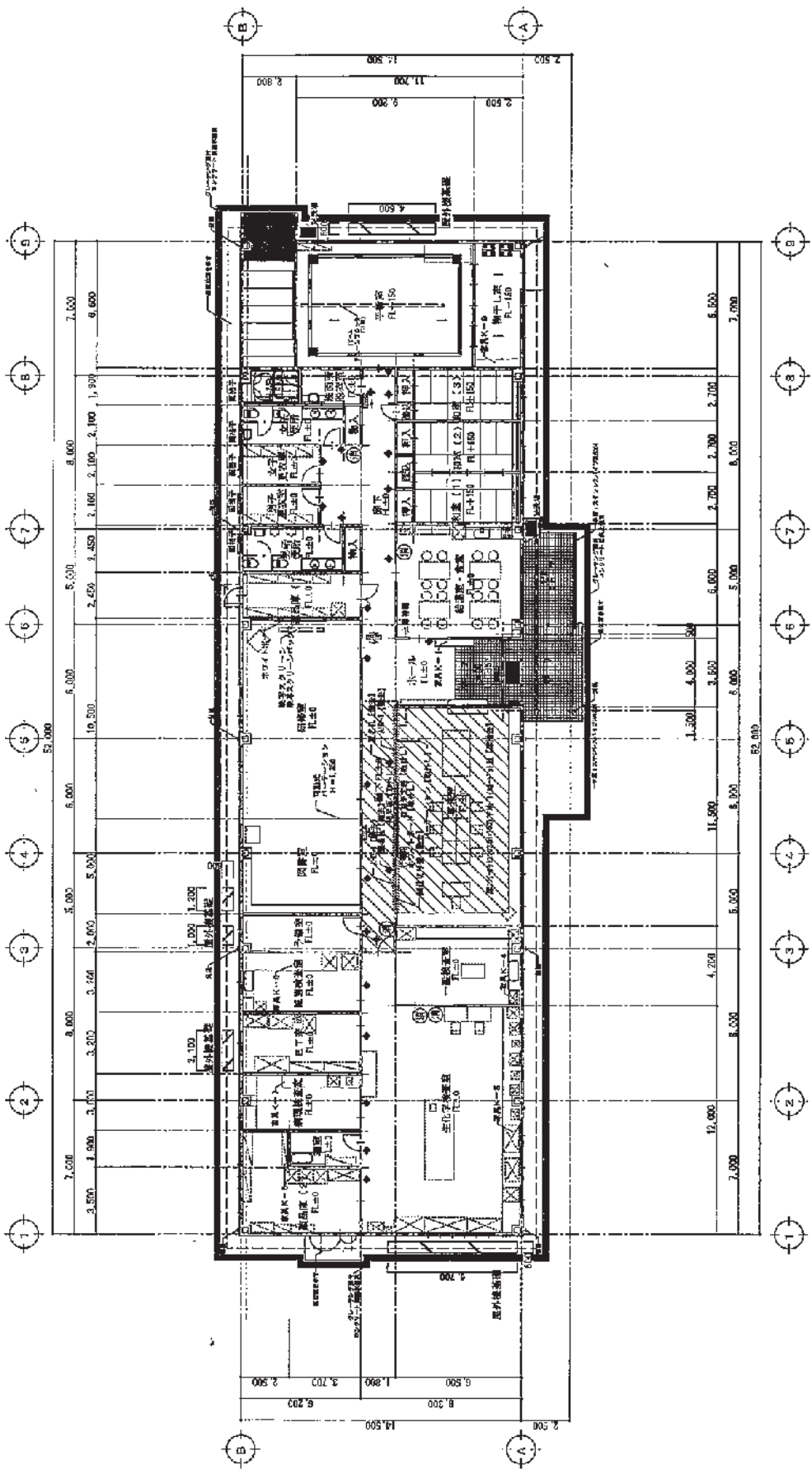
現状平面図 S=1:150
